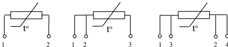
Приложение 2. Условное обозначение схемы внутренних соединений по ГОСТ 6651
