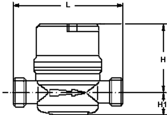
ПРИЛОЖЕНИЕ 1 Габаритные и присоединительные размеры счетчика воды одноструйного «ПУЛЬСАР»
