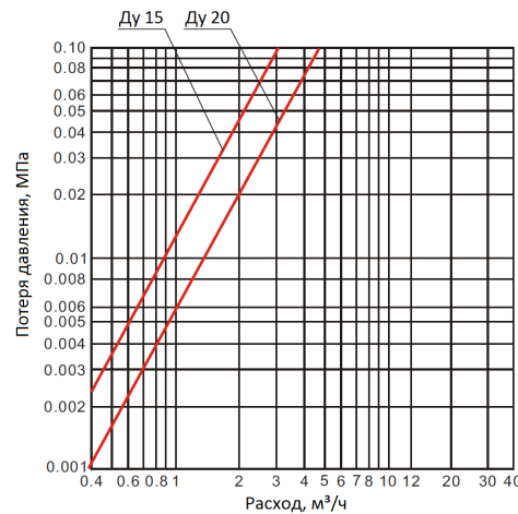
ПРИЛОЖЕНИЕ 2 Диаграмма потери давления
